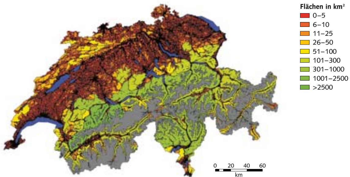
Zerschneidungskarte der Schweiz für das Jahr 2002 für «Landflächen unterhalb 2100 m» (ZG 4)
