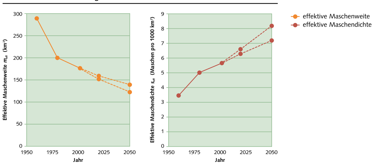
Erwartete Werte der effektiven Maschenweite und der effektiven Maschendichte in der Schweiz für die Jahre 2020 und 2050 bei anhaltendem Trend der Landschaftszerschneidung
