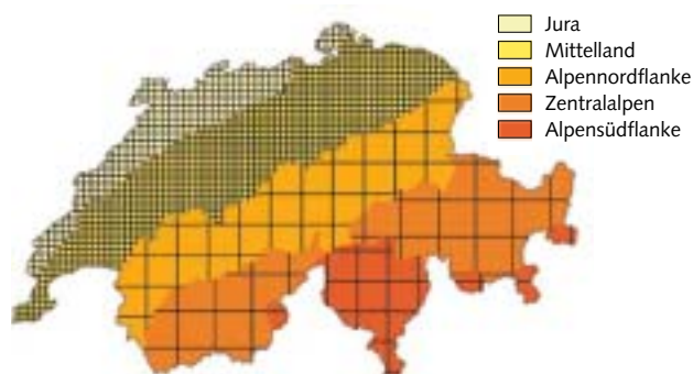
Schematische Darstellung der effektiven Maschenweite in den fünf Grossräumen im Jahr 2002 für «Landflächen unterhalb 2100 m» (ZG 4) A 10
